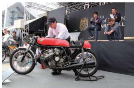
'50~'60年代当時、世界の2輪レースの頂点と目されていたマン島TTをはじめとするロードレース世界選手権に挑戦し、勝利した日本製マシン。そのエンジン始動パフォーマンスが行われ、迫力のサウンドをお楽しみいただきました。
